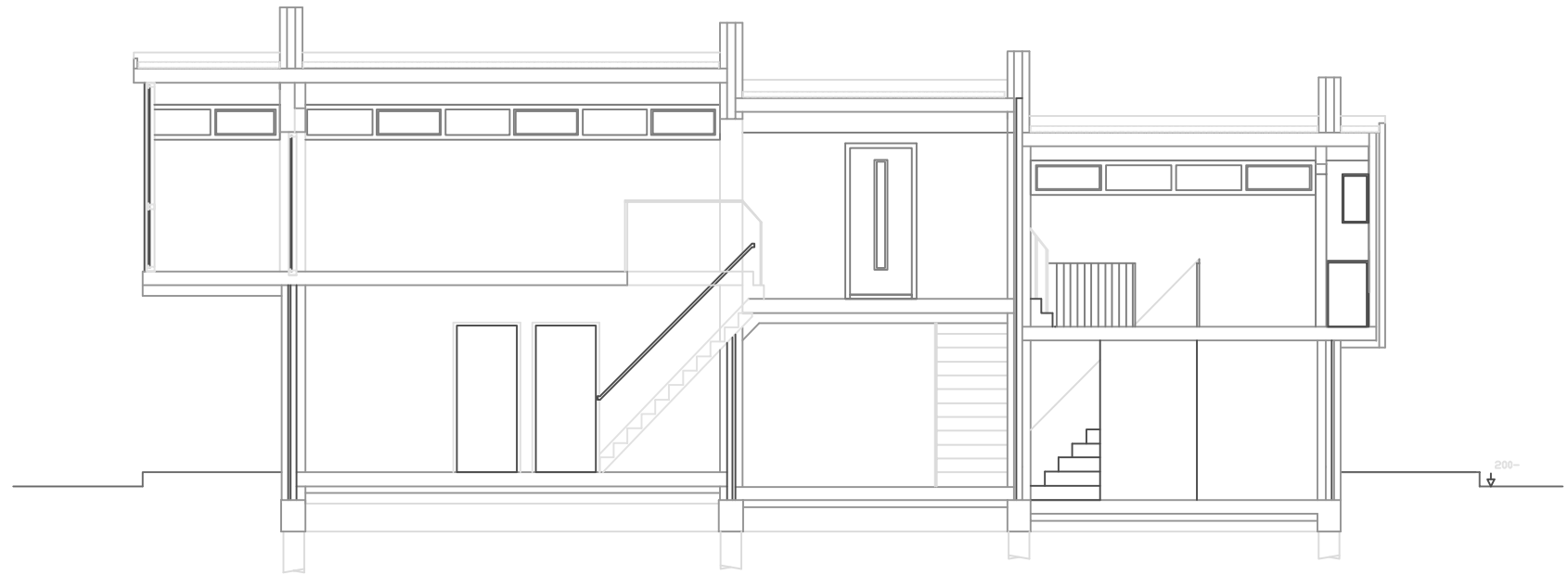
Doorsnede A-A
